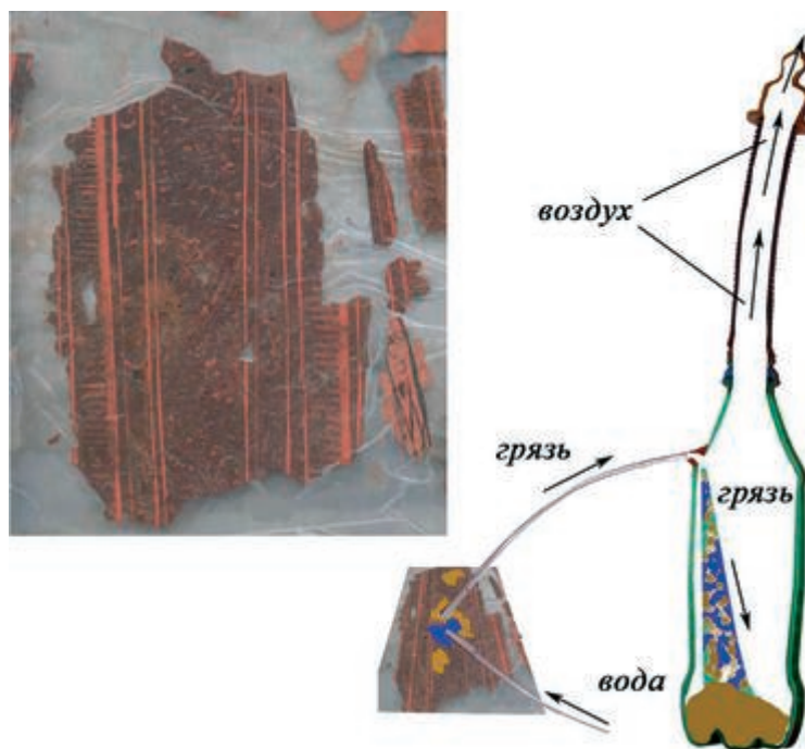
Рис. 5. СХЕМА ПРОЦЕССА ПРОМЫВКИ ФРАГМЕНТОВ ЛАКОВОЙ РОСПИСИ ИЗ СКЛЕПА 720
